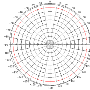
2.4GHz H面
