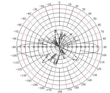
5GHz E面
