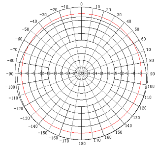
5GHz H面
