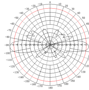
2.4GHz E面
