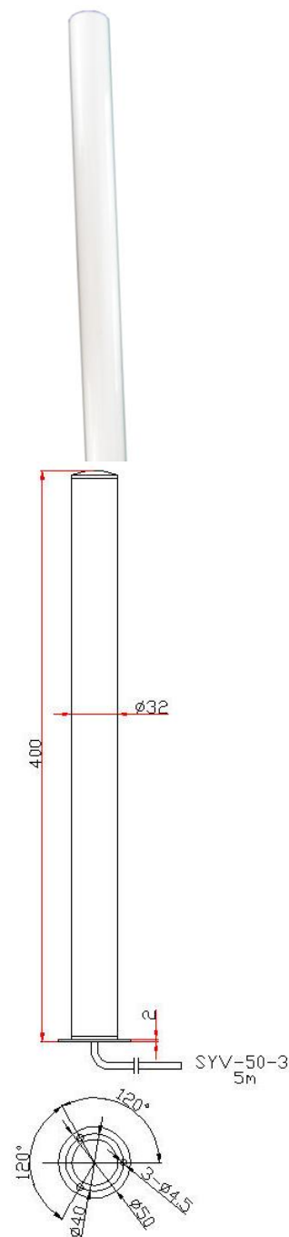
外形尺寸图
