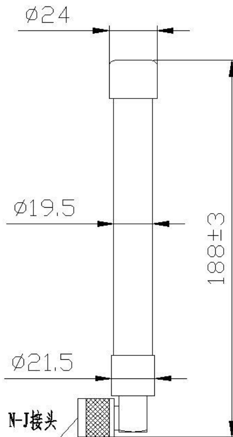
产品尺寸图
