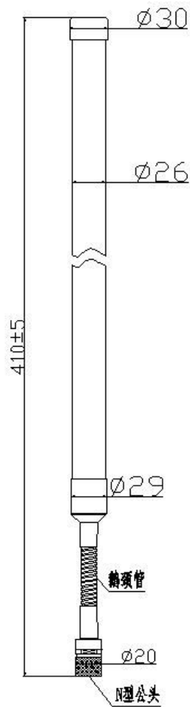
产品外形尺寸图
