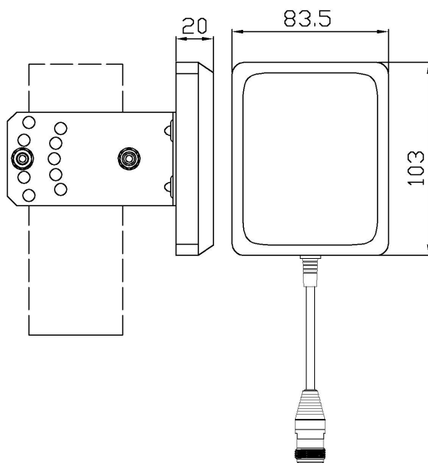
安装图
