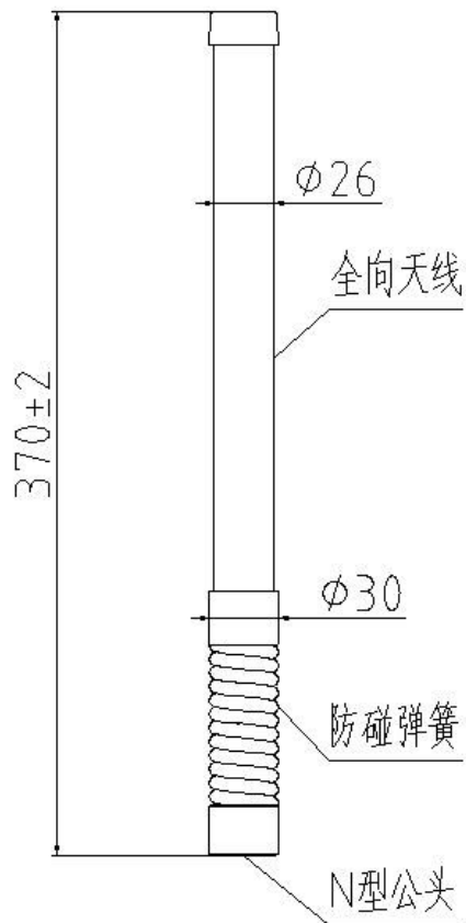
产品外形尺寸图
